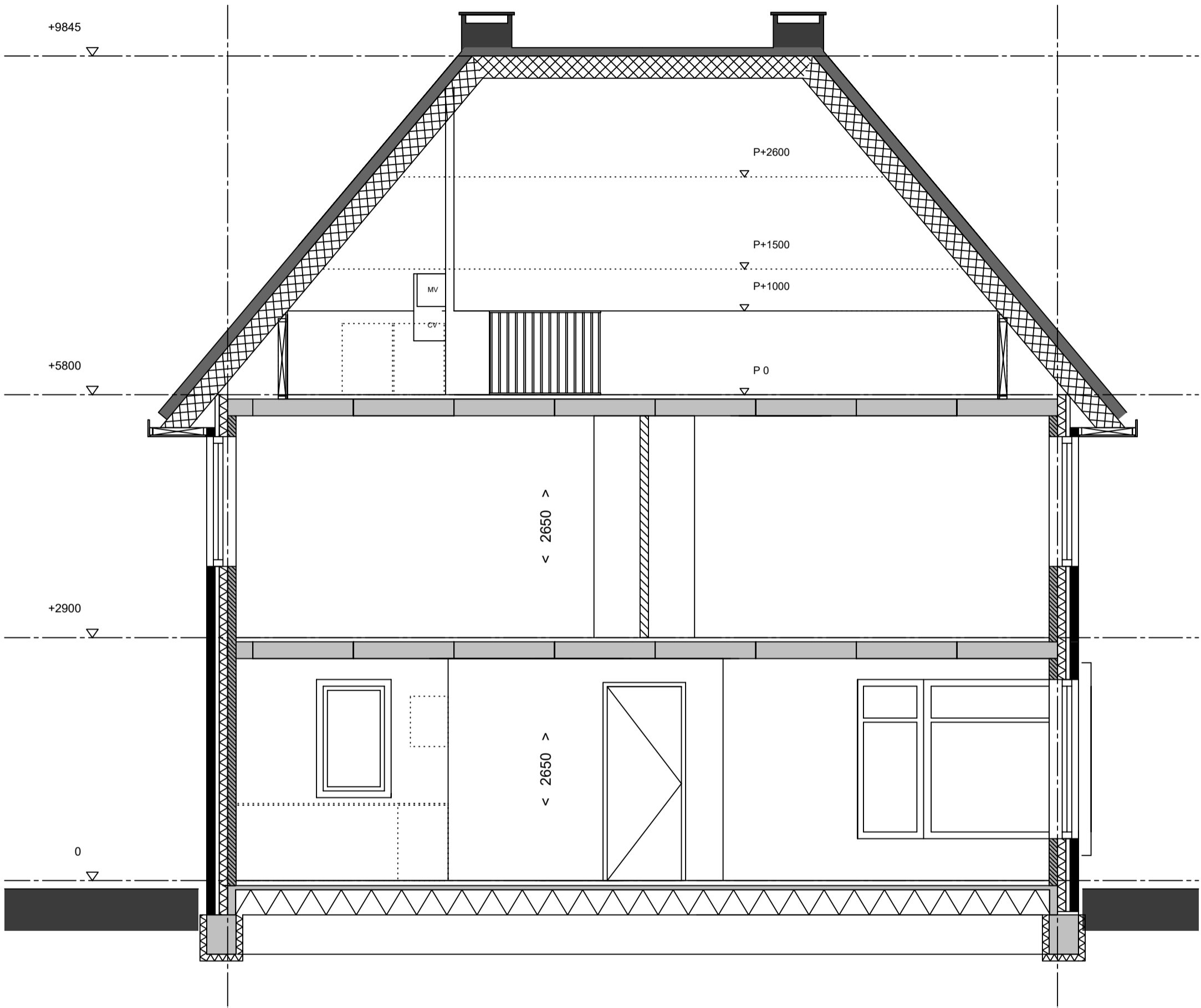
Doorsnede
